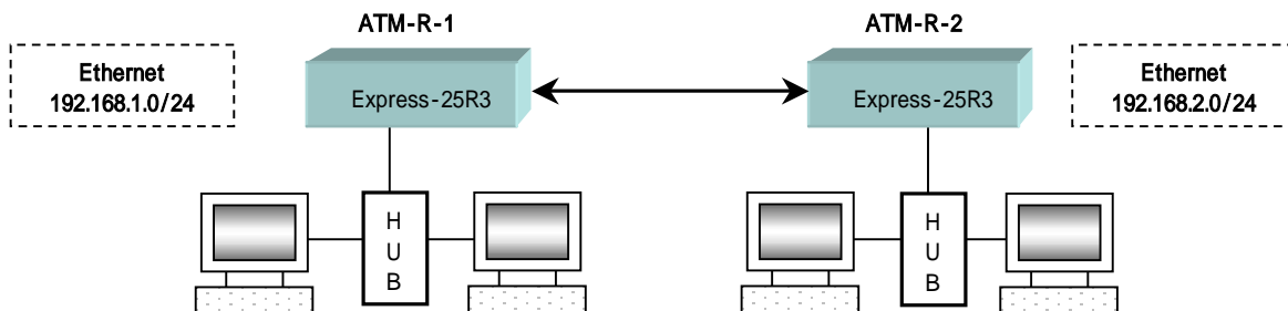
図 2.3.17.1 : デフォルトゲートウェイ設定できないホストの LAN 間接続
