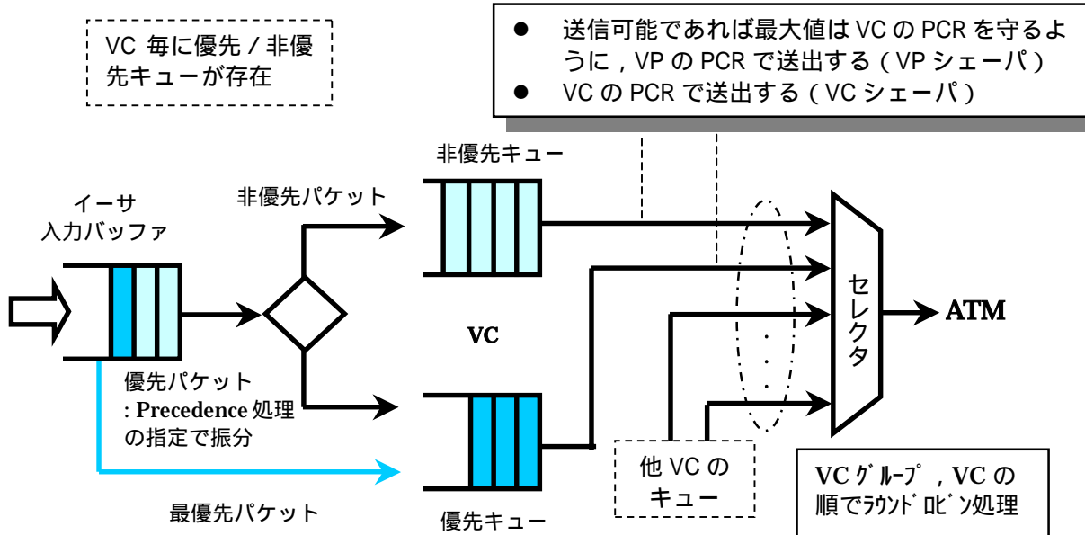
図2.3.15.1: パケットの優先制御
